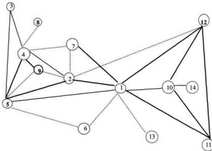
Значимые связи в коэффициентах Райского (R) [см. 5]
