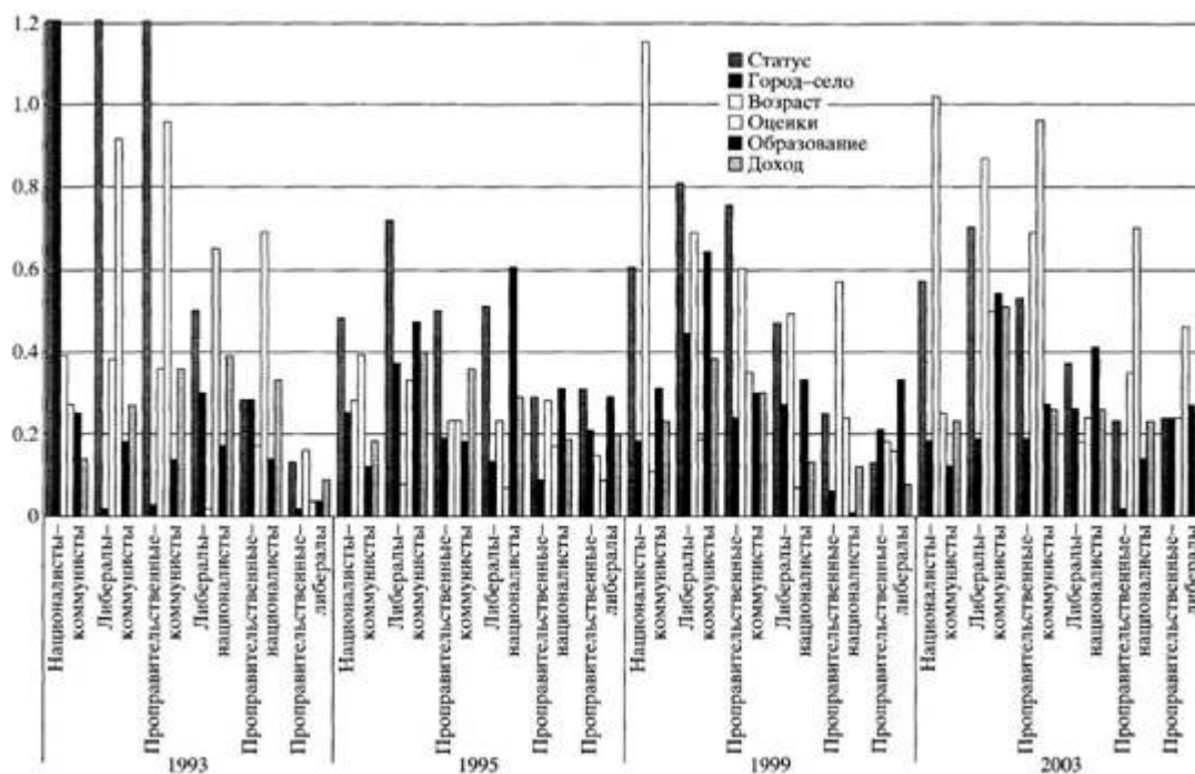
Диаграмма. Иллюстрация каппа-индексов размежеваний между парами партийных семей.
